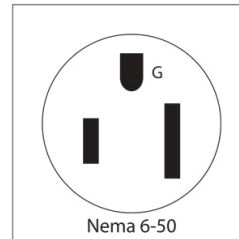
Nema 6-50
