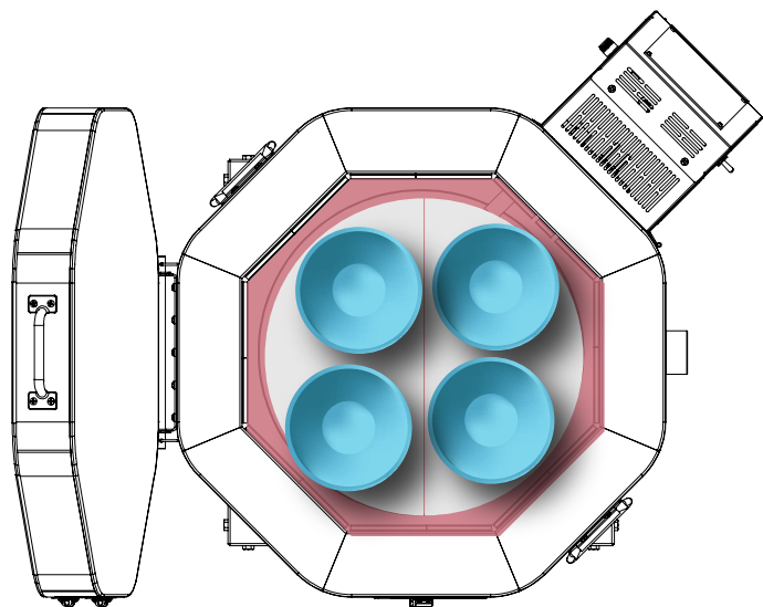
EASY-FIRE e18T-3 TOP VIEW
